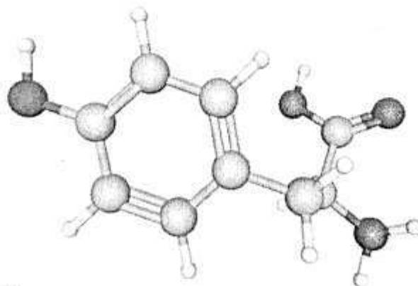
Tyrosine
