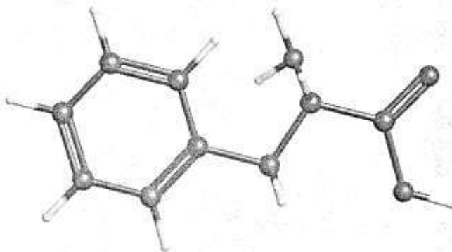
Tyrosine
